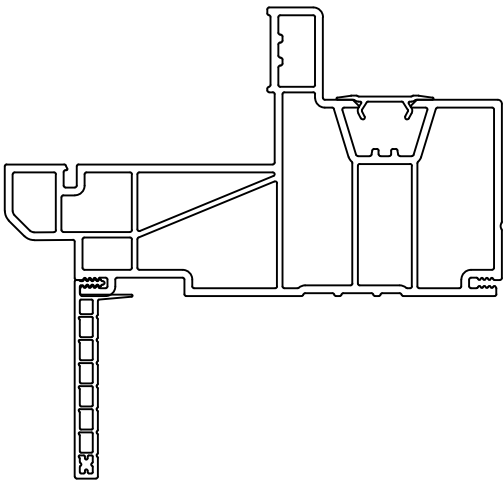
2" FLUSH FIN
