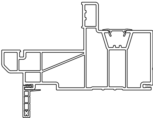
1" FLUSH FIN
