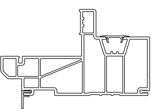
1/2" FLUSH FIN
